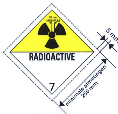
Groot etiket voor radioactieve stoffen van klasse 7
